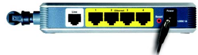
Figure 4-3 : Connexion de l'alimentation
